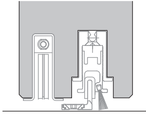
Guide au sol avec joint de fond (pour une meilleure isolation phonique)
