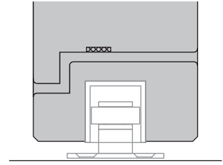
Guide au sol avec porte de service
