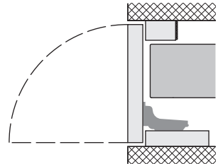
Raccord au mur du côté ouverture avec trappe (porte coulissante ouverte)
