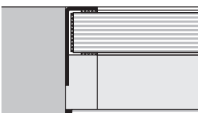
Angle unilatéral en acier inoxydable avec verre de sécurité trempé à fleur sur le côté arrière
