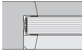
Unilatéral en feuilure
