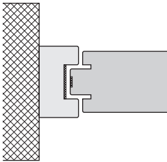
Profilé de butée sur le mur
