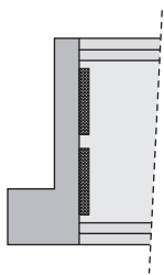
Modèle de chants en feuilure
