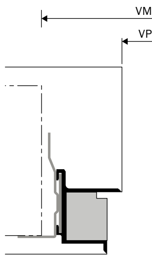
Huisserie à fleur de mur, masquée, ouverte vers l'extérieur
