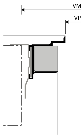
Huisserie à fleur de mur, masquée, ouverte vers l'intérieur
