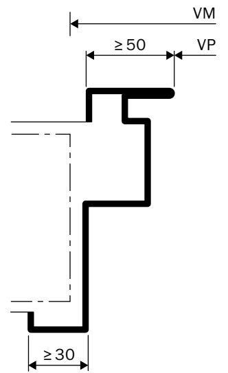
Huisserie en acier ouverture vers l'intérieur
