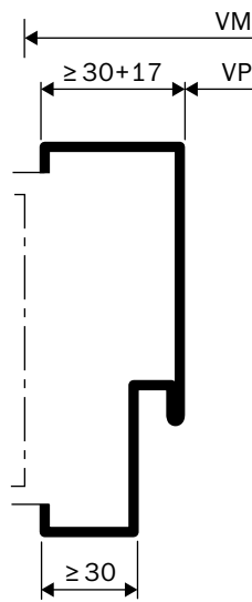
Huisserie enveloppante symétrique
