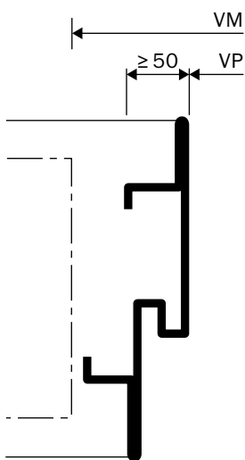
Huisserie design (sans miroir)
