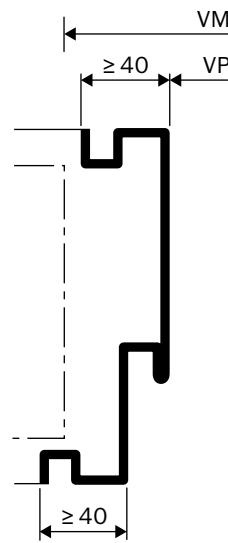
Huisserie avec joint d'ombre
