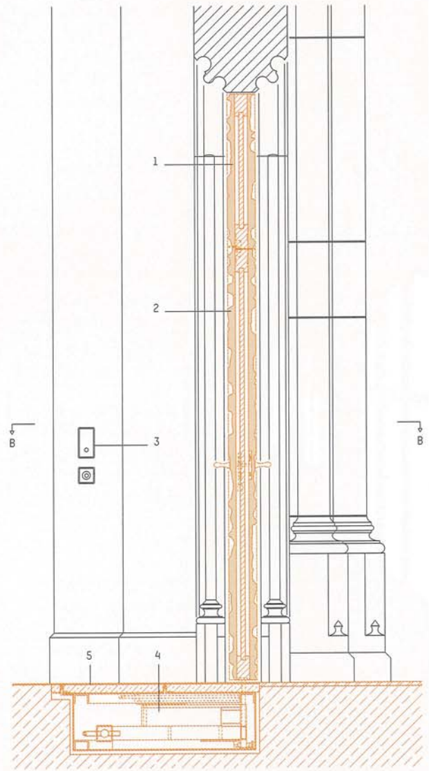
Vertikalschnitt Kriteriumstür M 1:25
