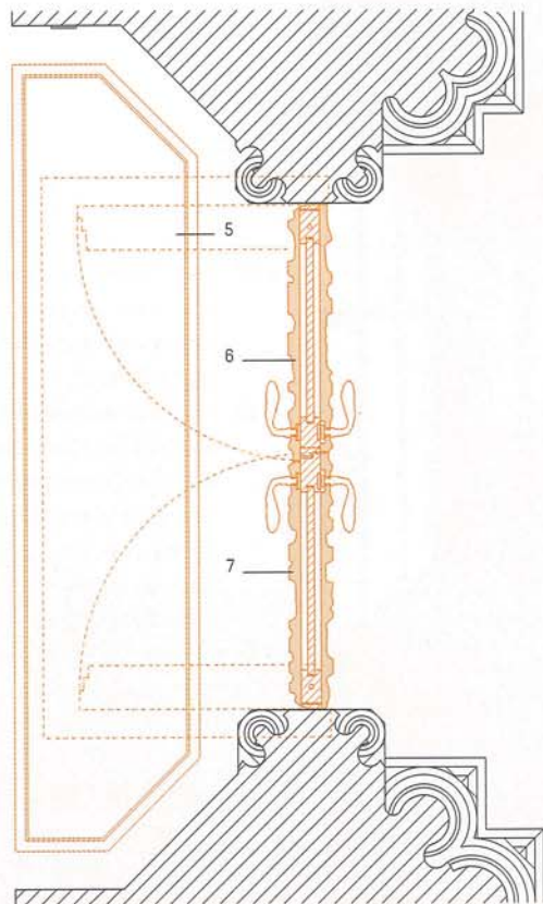
Horizontalschnitt Kriteriumstür [B-B] M 1:25
