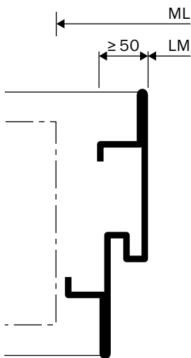
Designzarge (ohne Spiegel)
