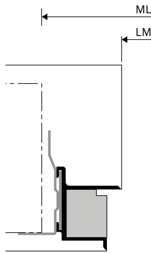
Zarge wandbündig verdeckt, auswärts öffnend
