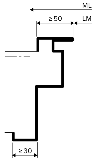
Stahlzarge nach innen öffnend
