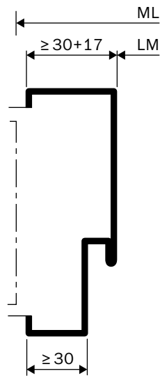
Umfassungszarge spiegelgleich
