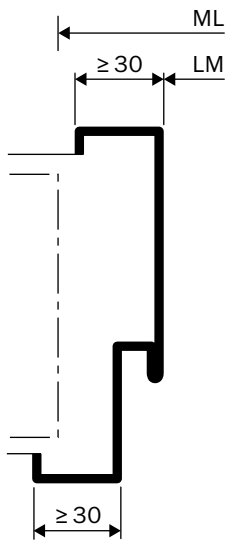
Umfassungszarge
