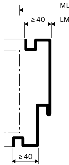
Schattennut-Zarge
