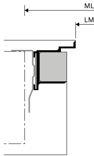
Zarge wandbündig verdeckt, einwärts öffnend
