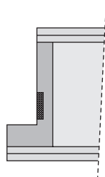
Kantenführung gefälzt
