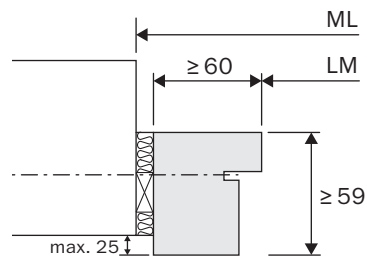
Holzblockrahmen vorstehend
