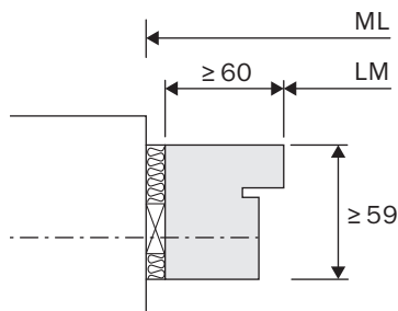
Holzblockrahmen
