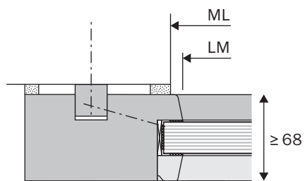
auf Wand mit Nutleiste
