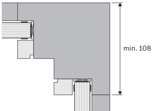
Brandschutzverglasung EI60 Innenanwendung
