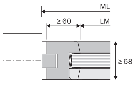
zwischen Wand mit Nutleiste (max. 2-seitig möglich)
