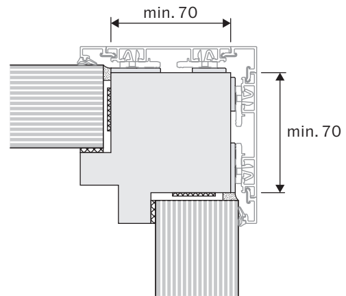
Brandschutzverglasung EI30 Aussenanwendung
