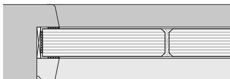
Brandschutzverglasung EI30 mit Silikonfuge, ohne Randemail
