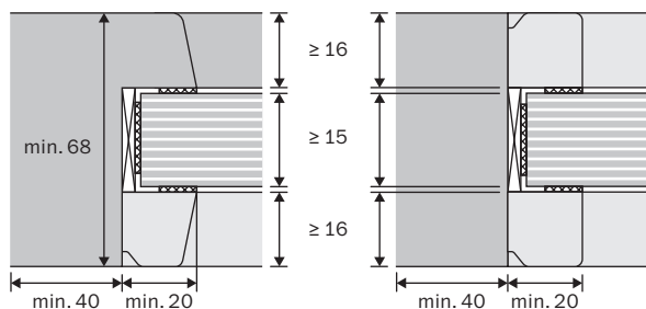
Glasstab einseitig
