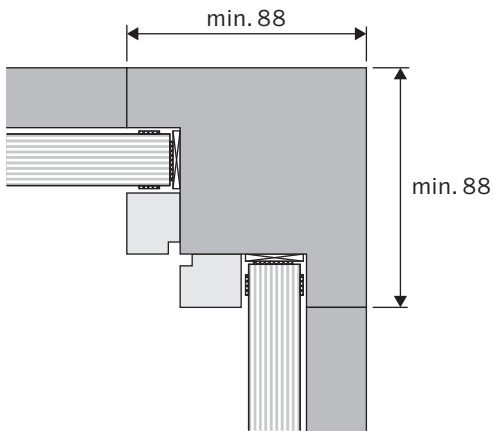
Brandschutzverglasung EI30 Innenanwendung
