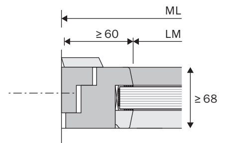
zwischen Wand mit Falzleiste
