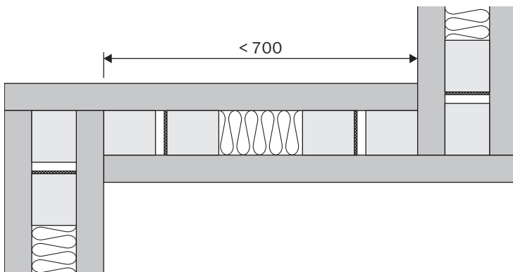
Brandschutztrennwand EI60 RF1 mit Deckellösung
