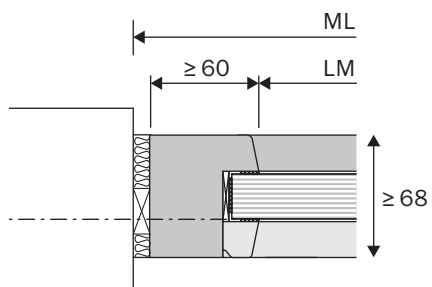
zwischen Wand direkt verschraubt
