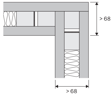
Brandschutztrennwand EI60 RF1
