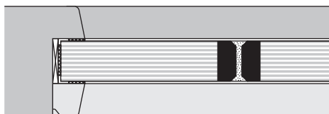
Brandschutzverglasung EI30 mit Silikonfuge, mit Randemail
