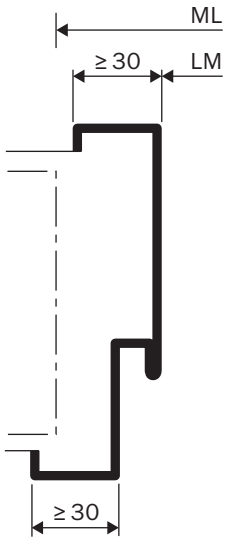
Umfassungszarge
